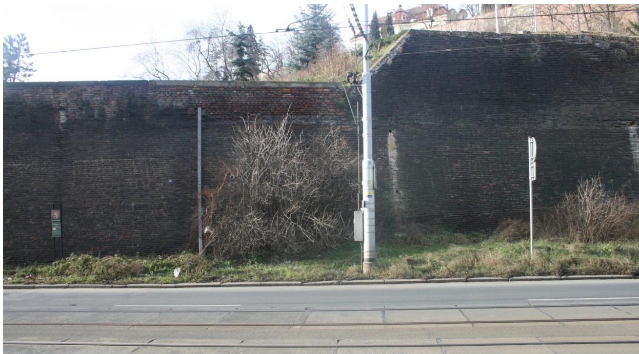
Pohled na střední část zdi 2B z nábrž.E.Beneše
